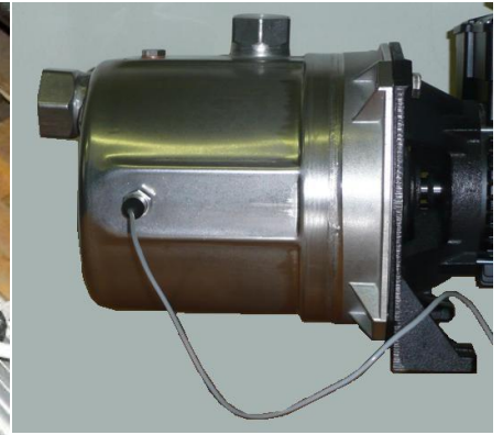
Obr 3: príklad montáže senzora na čerpadlo do plniaceho otvoru
